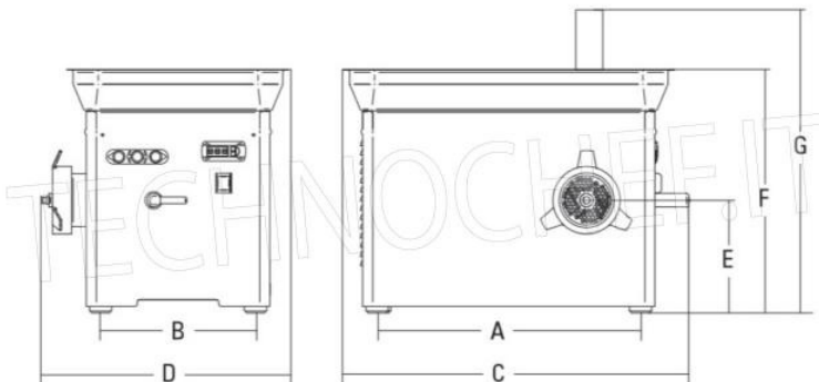
Dimensioni mm
