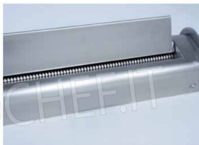
Tagliasfoglia inox con aggancio e sgancio rapido larghezza utile mm. 260, sponda di appoggio per facilitare l'imbocco sfoglia, ottenendo così una maggior produzione. (OPZIONALE)
